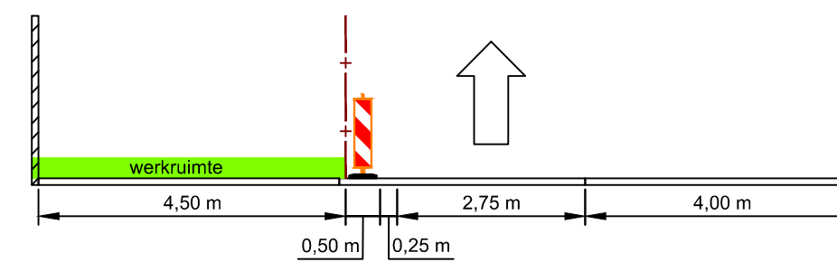
DOORSNEDE B SCHAAL 1:100
